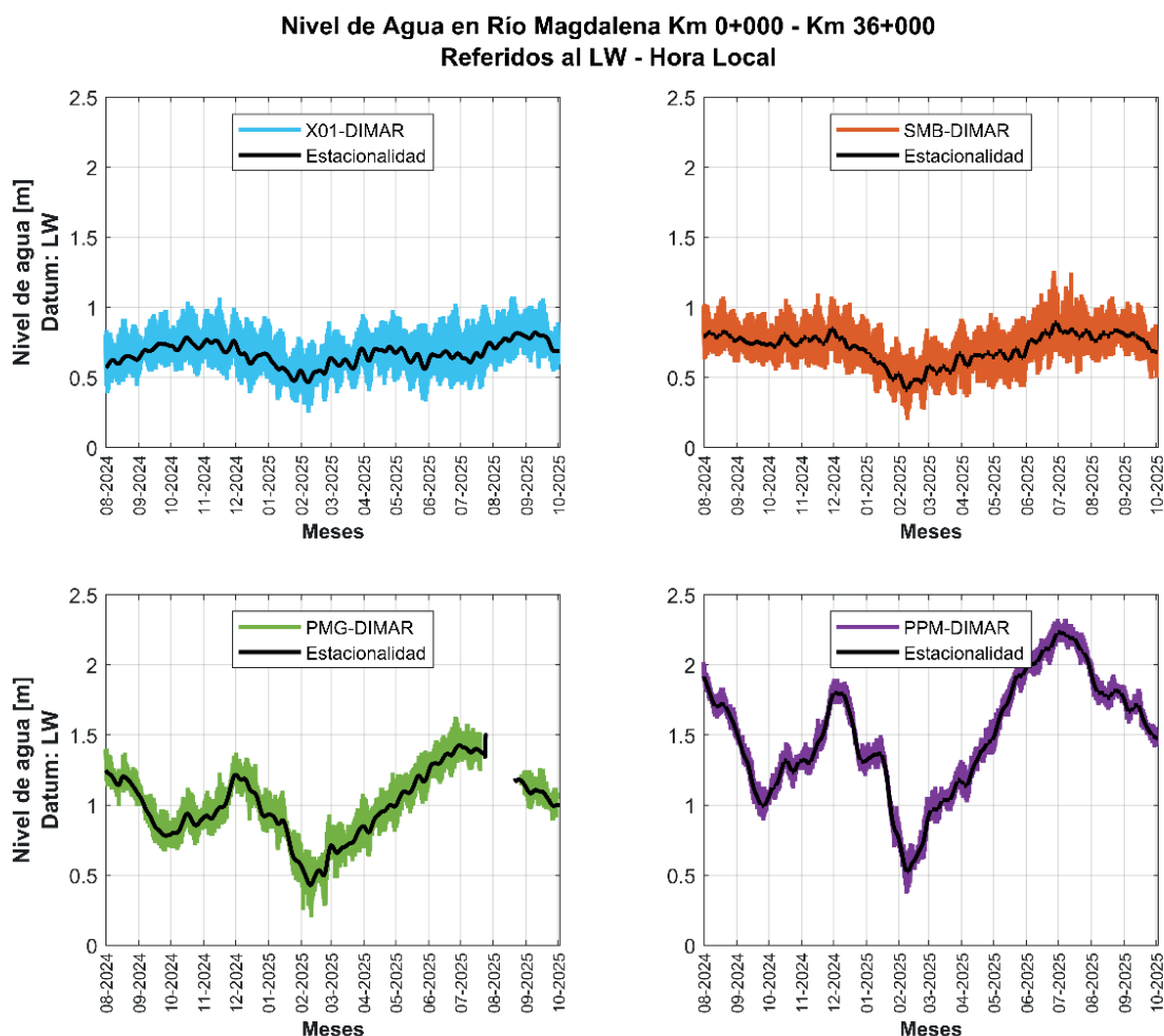
Figura 39. Serie temporal comportamiento niveles de agua y estacionalidad en el Río Magdalena (km 0 al km 36).
