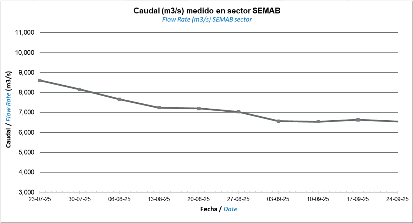
Figura 38. Evolución comportamiento caudal sección transversal km 8+500.
